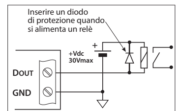
Collegamento tipico attivazione relé allarme
