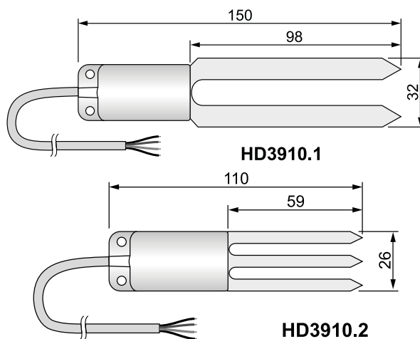
Fig. 1: dimensioni (mm)
