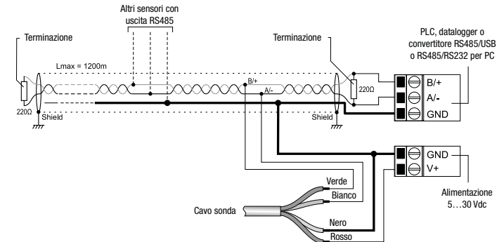
Fig. 3: connessione RS485
