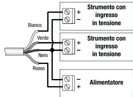
Fig. 4: connessione uscite analogiche
