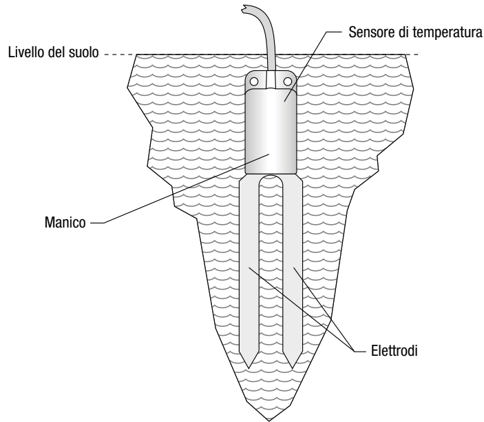
Fig. 2: installazione
