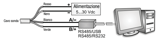
Fig. 5: collegamento al PC
