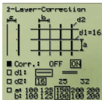
Esempio schermata SCANLOG
