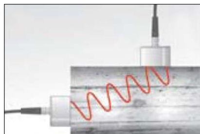
Trasmissione semidiretta
